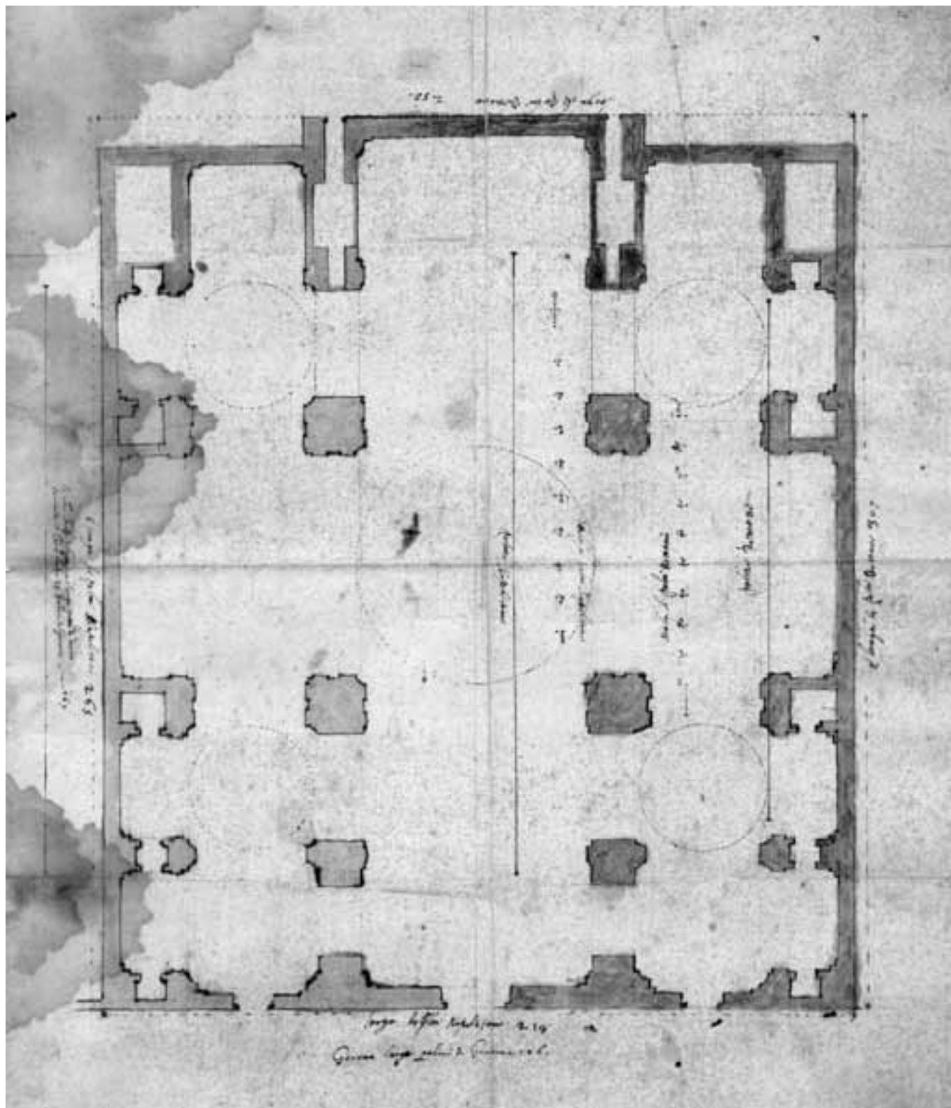
120. Neapel, Gesù Nuovo, Planaufnahme, um 1600.
