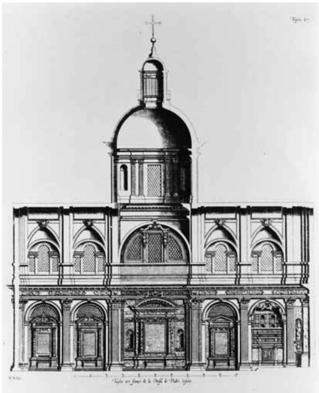
118. Genua, SS. Ambrogio e Andrea, Längsschnitt (Kupferstich).
